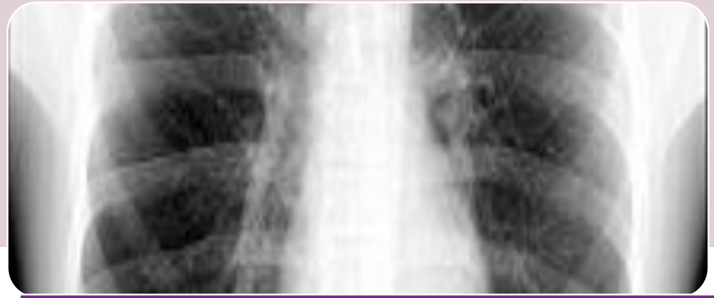
Kostra trupu
