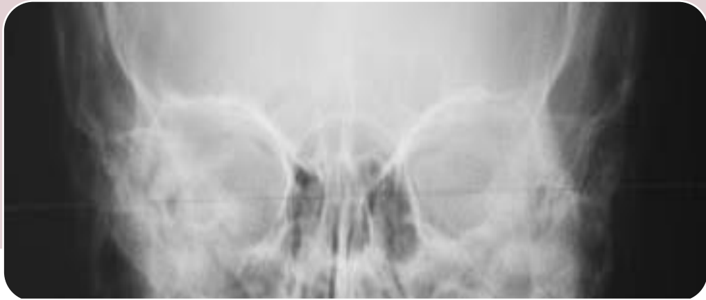
Kostra hlavy
